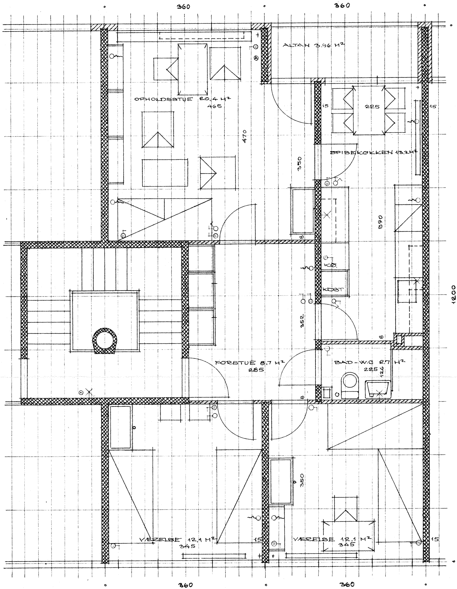
HØBLERINGSPLAN 1 MÅL 1:50 LEJLIGHEDSTYPE 6 - 3 VÆR. - 83,88 M 2 EKSKL. ALTAN BLOK 21, 22 OG 23
