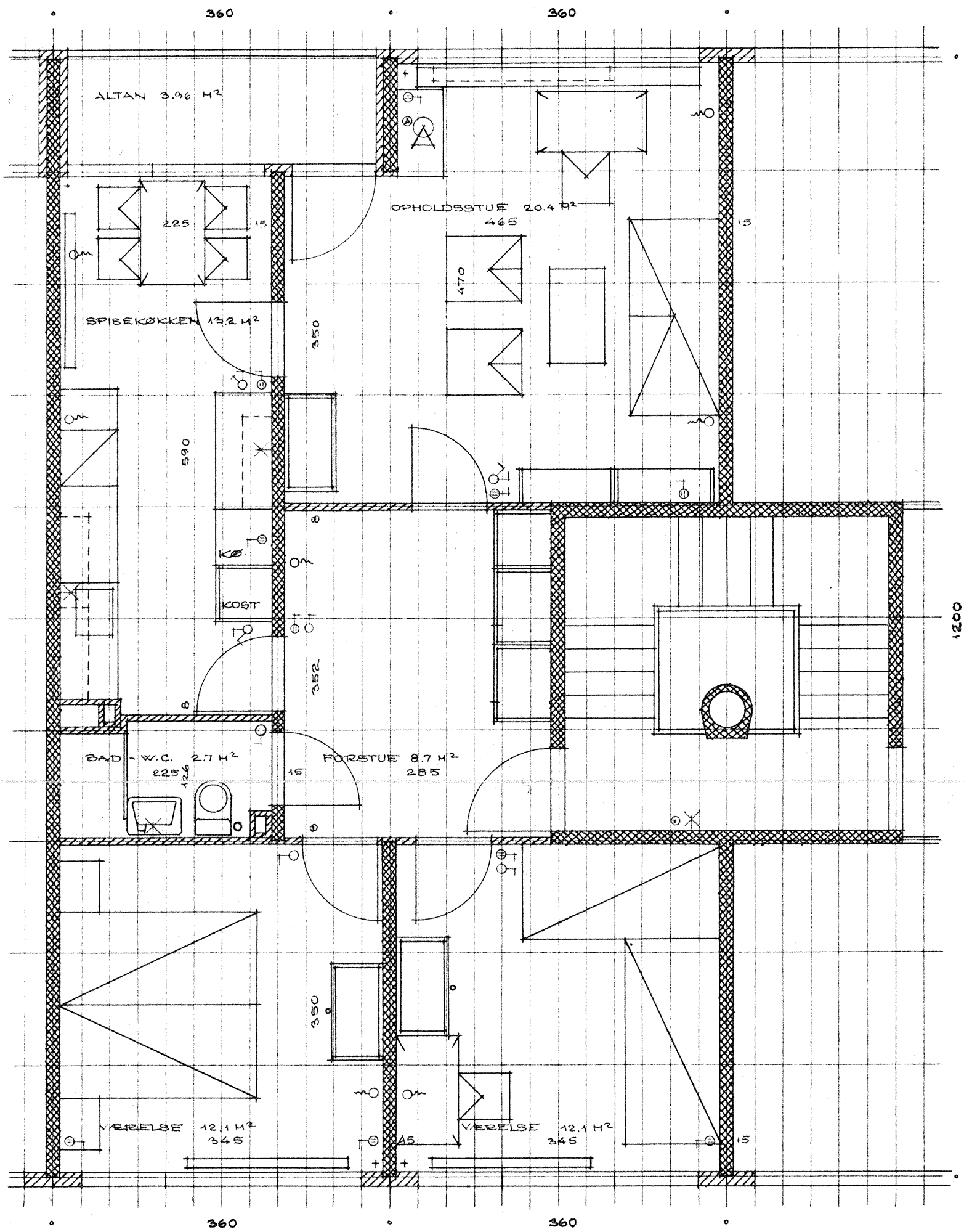
MØBLERINGSPLAN 1 MÅL 1:50 LEJLIGHEDSTYPE 5 - 3 VER - 83.88 M 2 ESKL. ALTAN BLOK 21, 22 OG 23
