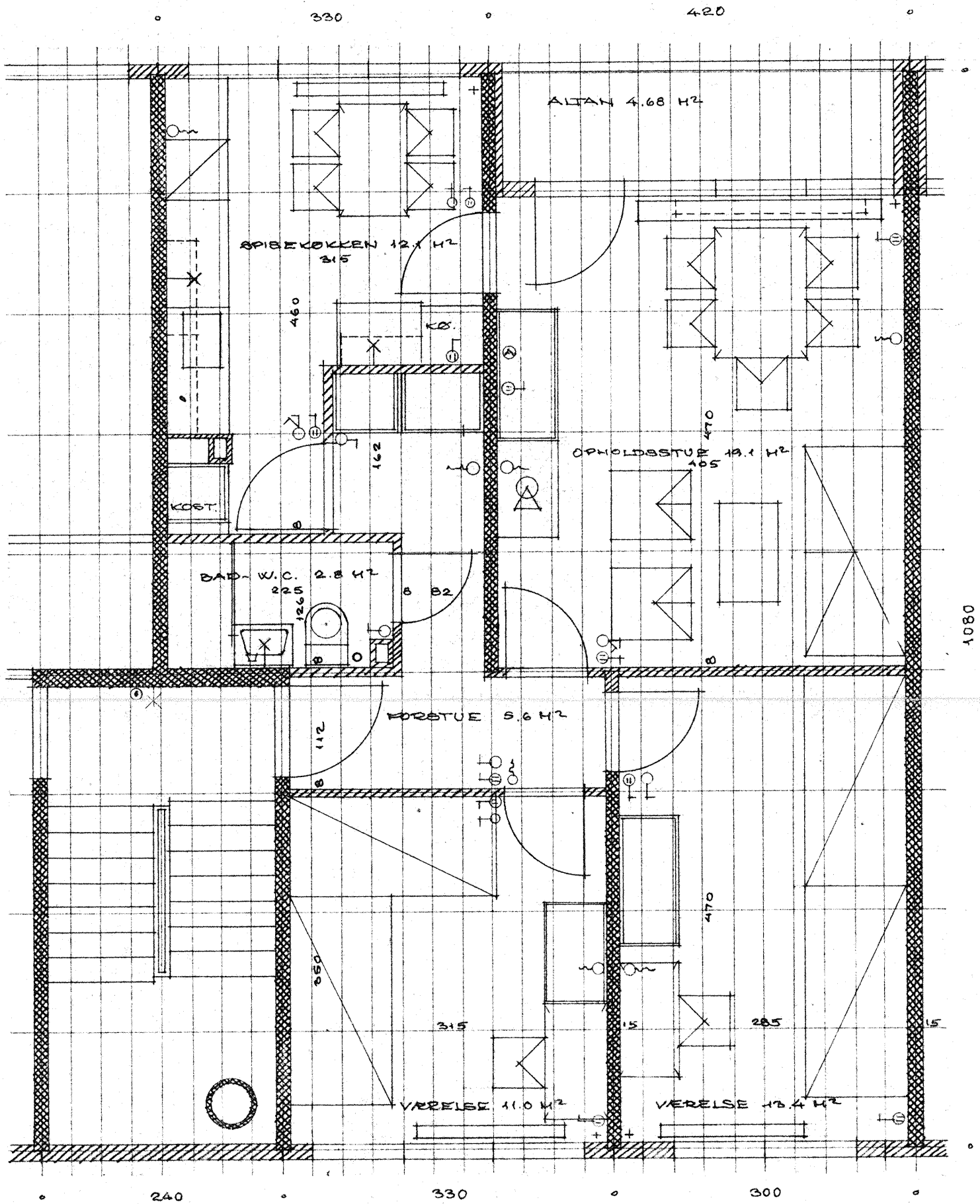
MØBLERINGSPLAN I MÅL 1:50 LEJLIGHEDSTYPER 4 - 3 VÆR. - 77.82 M 2 EKSKLUSIV ALTAN BLOK 13
