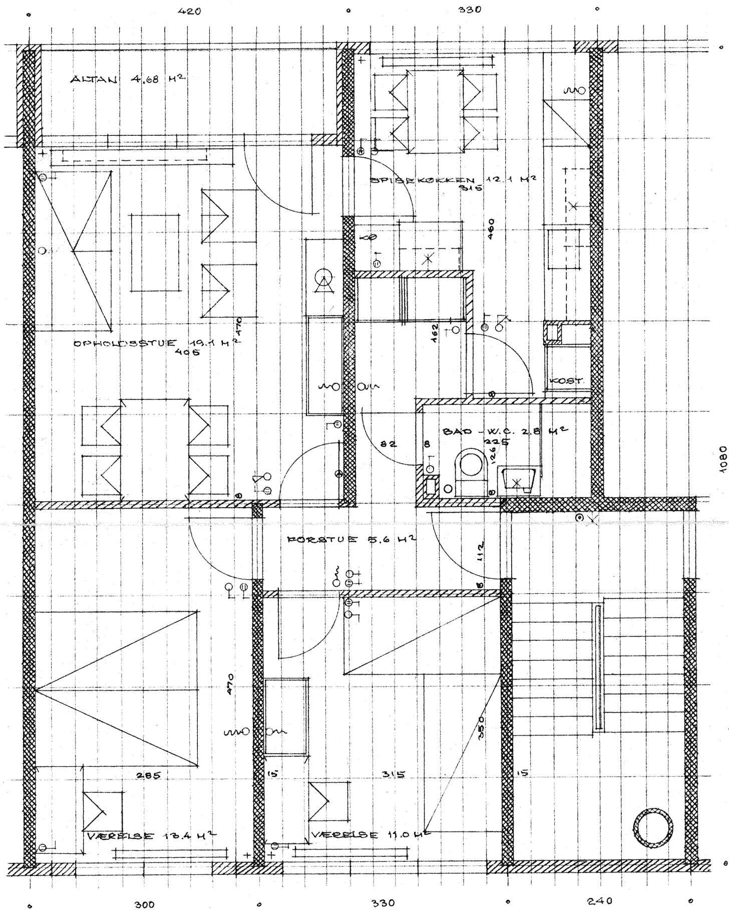
MØBLERINGSPLAN I MÅL 1:50 LEJLIGHEDSTYPE 3 - 3 VÆR. - 77.82 M 2 EKSKLUSIV ALTAN BLOK 13
