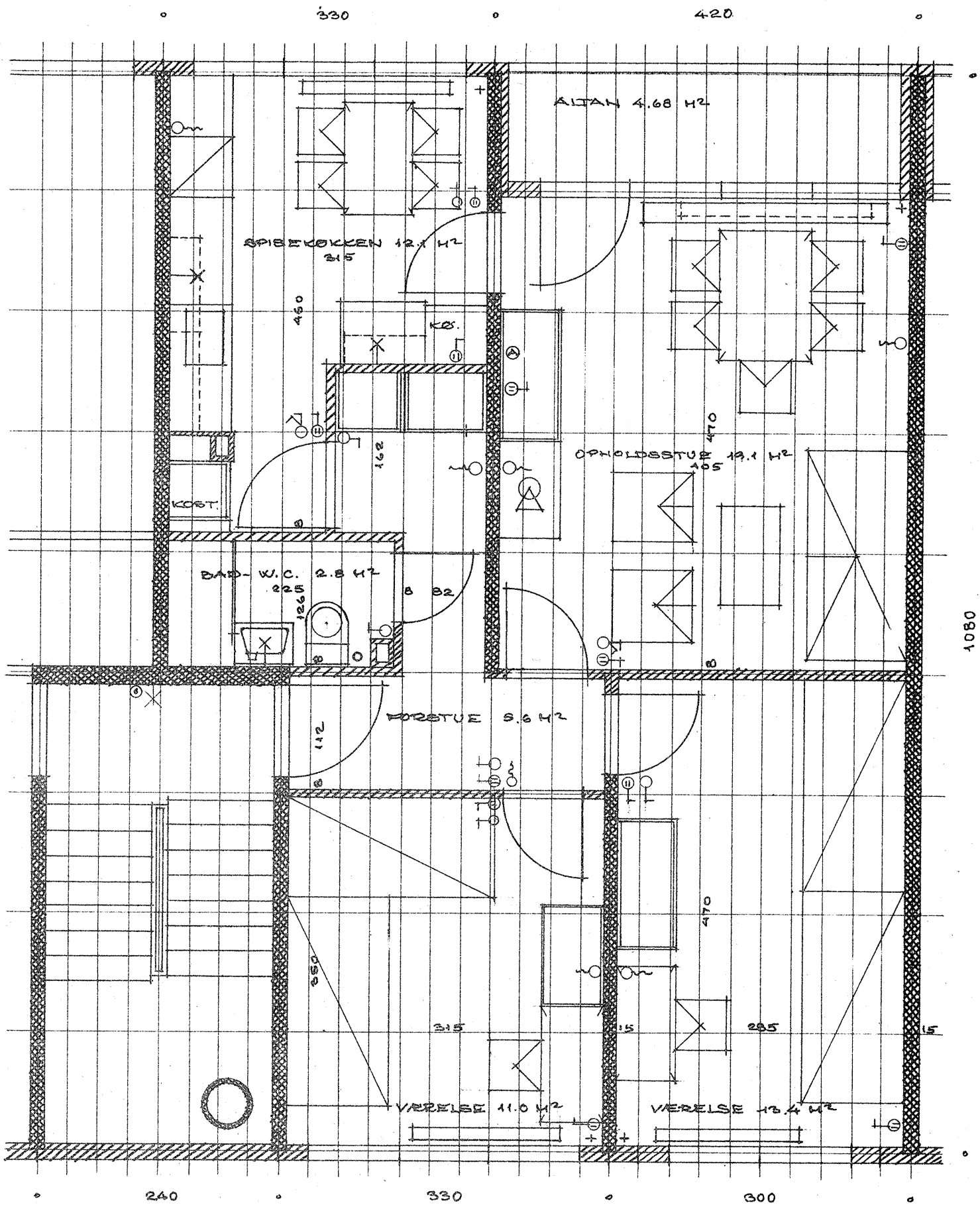
HØBLERINGSPLAN 1 MÅL 1:50 LEJLIGHEDSTYPE 4 - 3 VÆR. M. SPISEKØKKEN - 78,49 M 2 . BLOK 13
