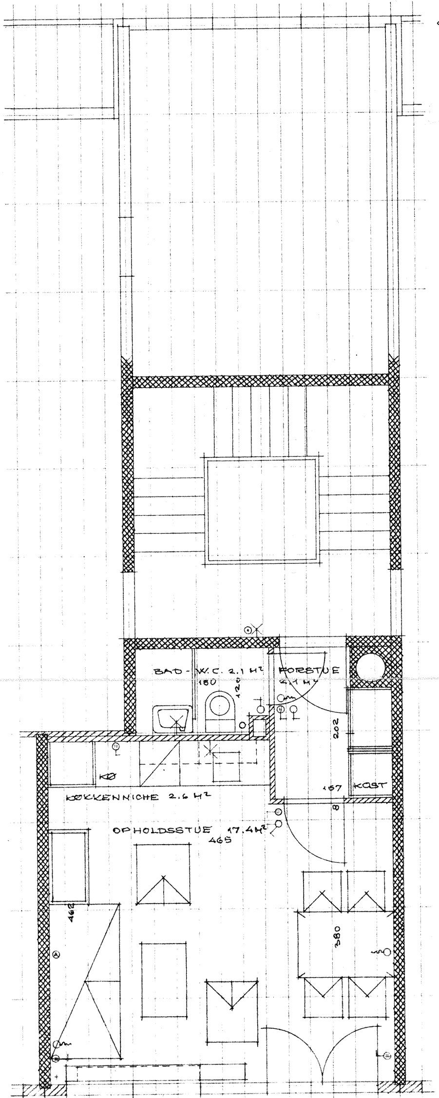
MØBLERINGSPLAN I MÅL 1:50 LEJLIGHEDSTYPE 11 - 1 VÆR. 31.93 M 2 BLOK 31 OG 32
