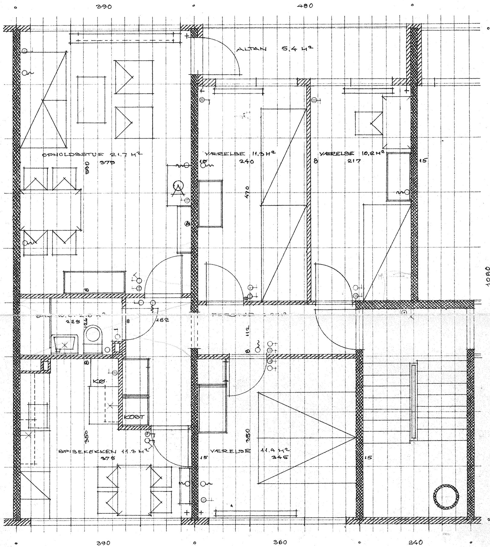
MØBLERINGSPLAN I MÅL 1:50 LEJLIGHEDSTYPE 1 - 4 VÆR. - 90,30 M 2 EKSKLUSIV ALTAN BLOK 11 OG 12
