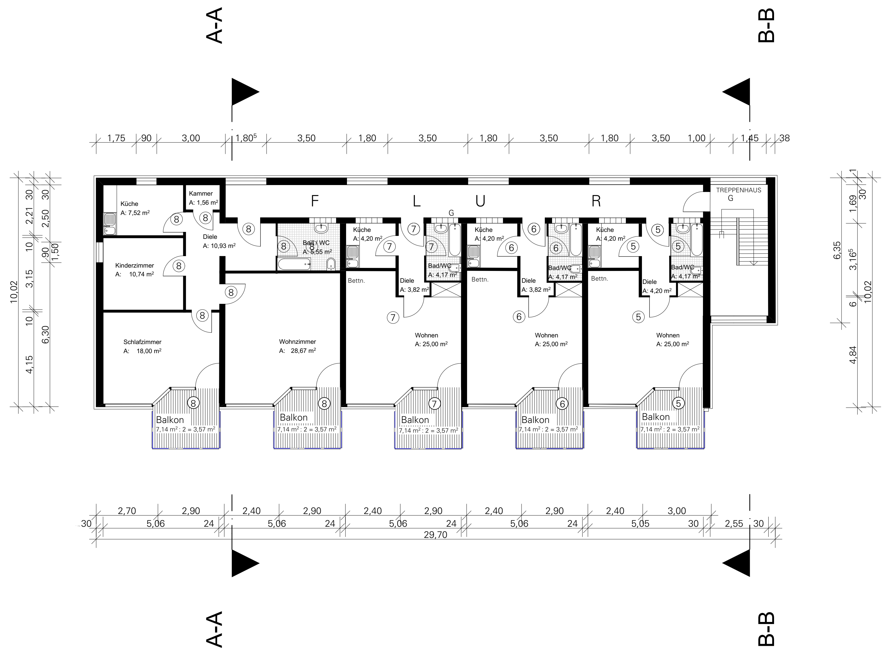
1. OBERGESCHOSS
