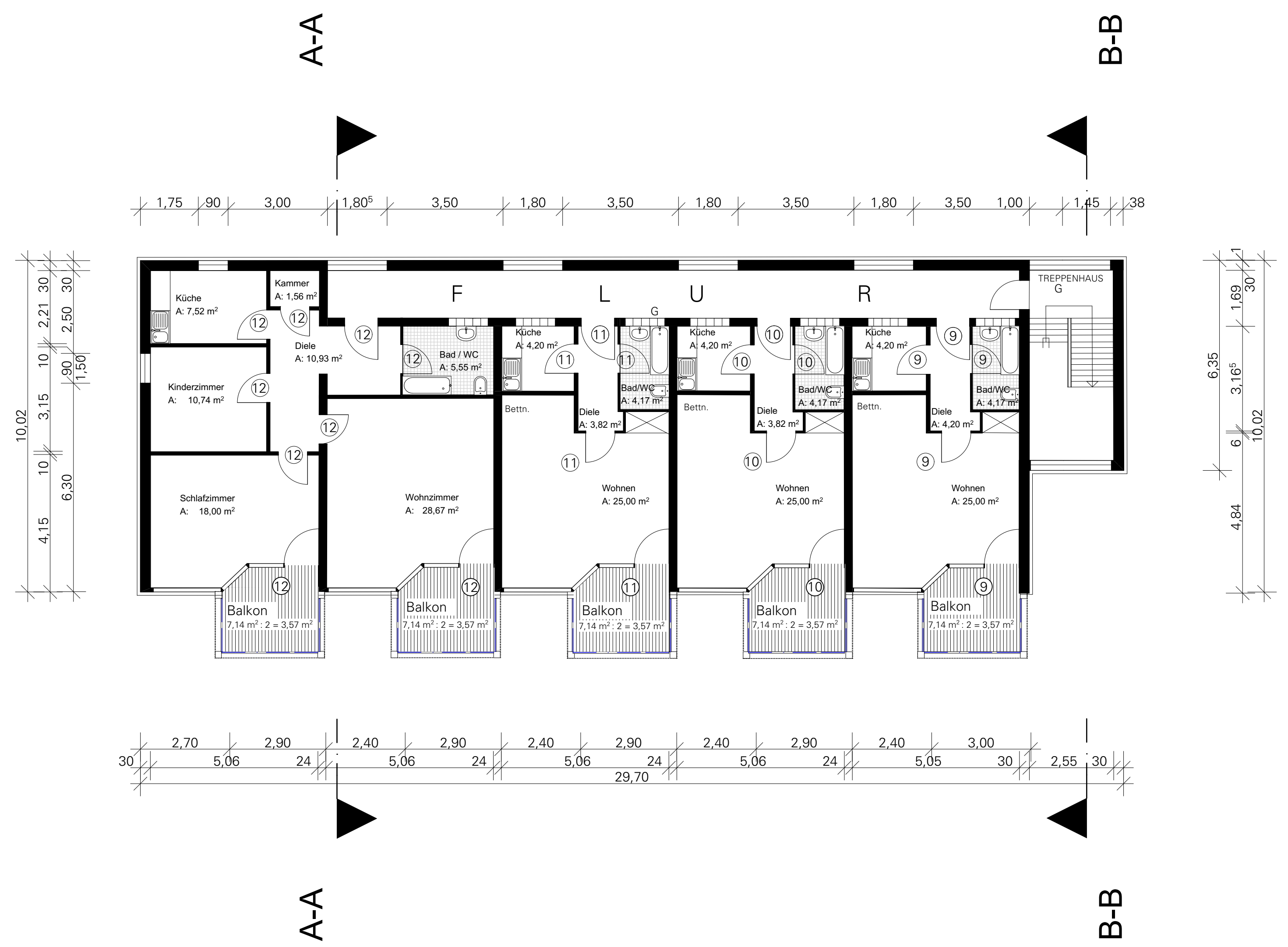
2. OBERGESCHOSS
