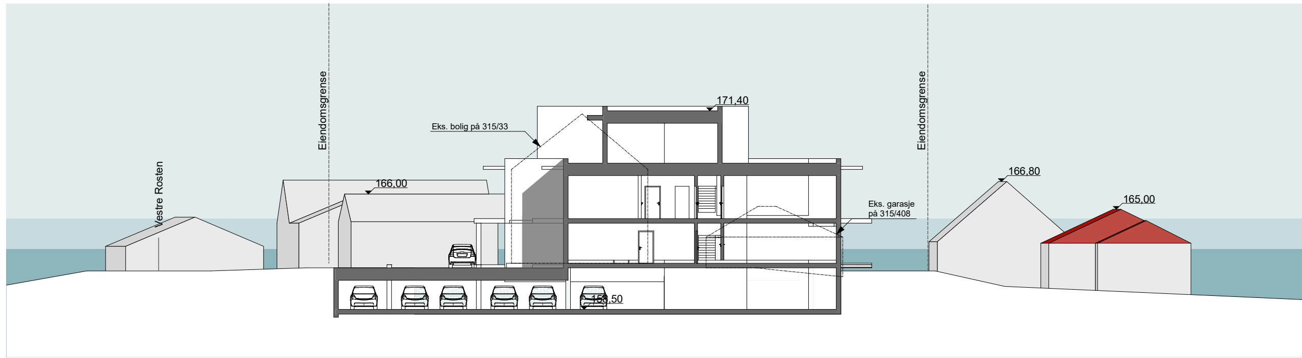
Snitt A-A
