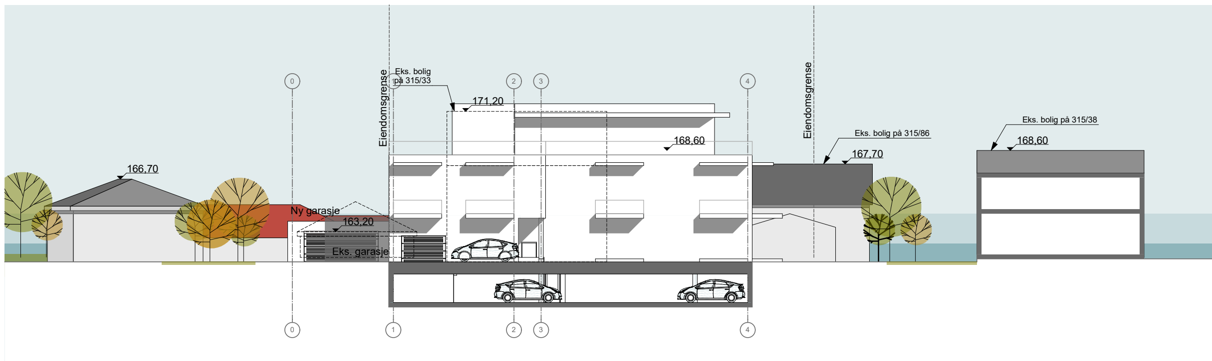
Snitt D-D
