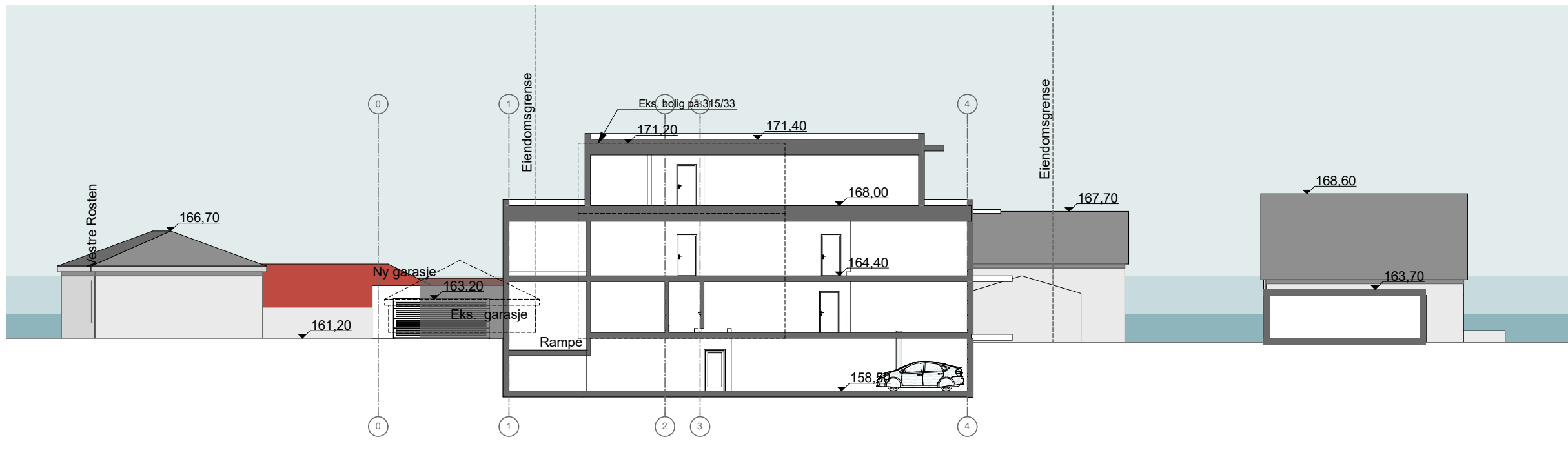
Snitt C-C
