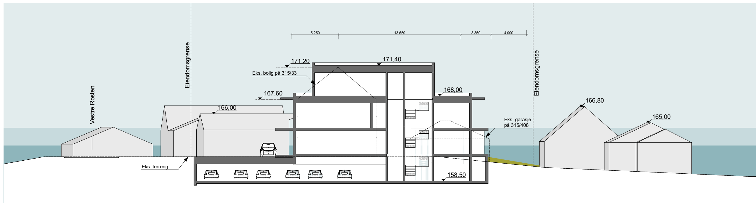
Snitt B-B
