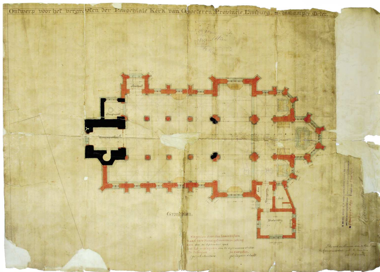
Ontwerptekening van de plattegrond van H. Martens en V. Lenertz (1904).
