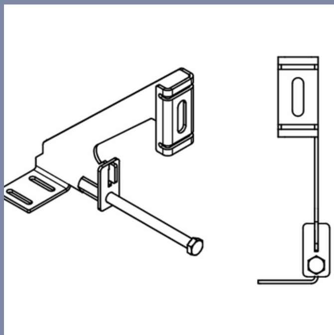
TSK-murkonsol type 1
