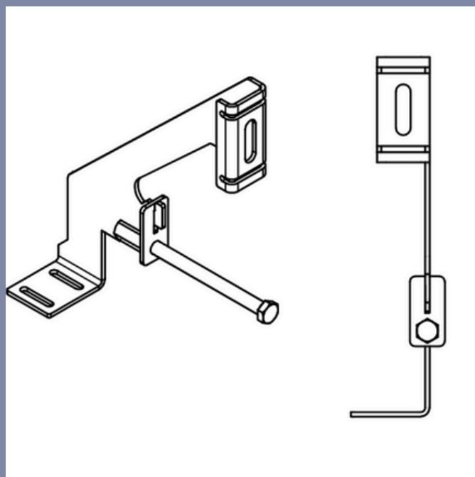
TSK-murkonsol type 2
