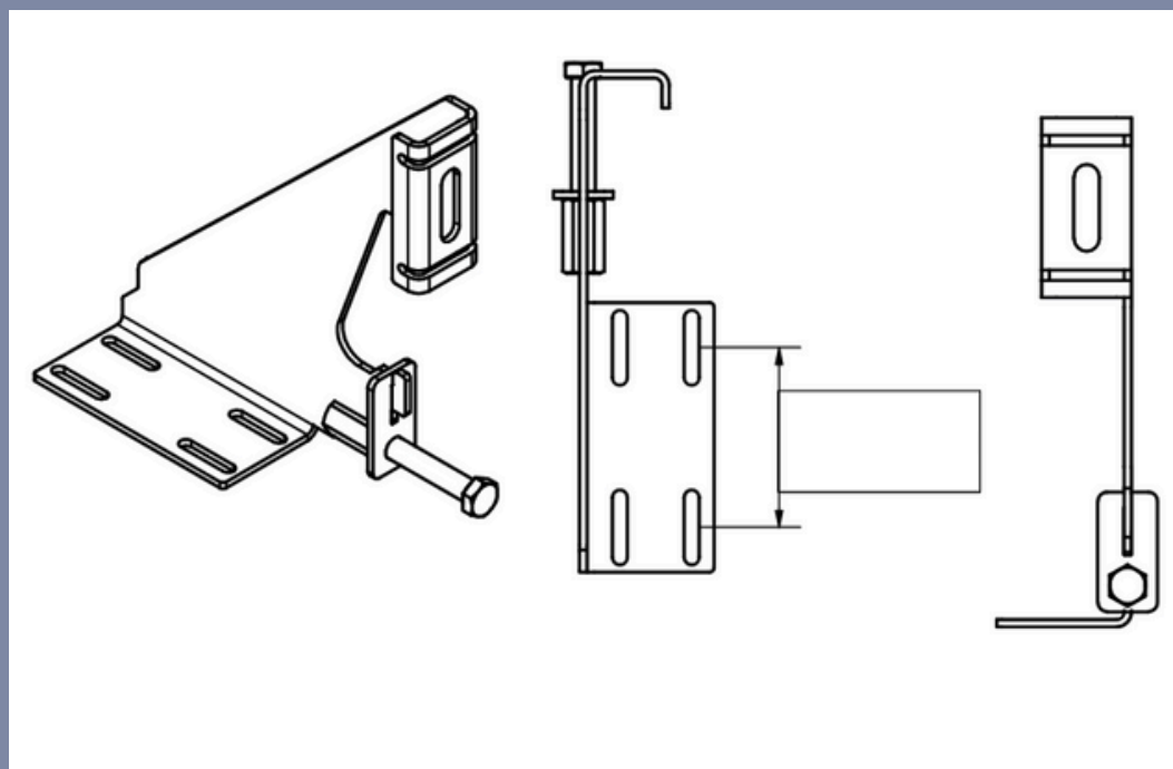
TSK-murkonsol type 4
