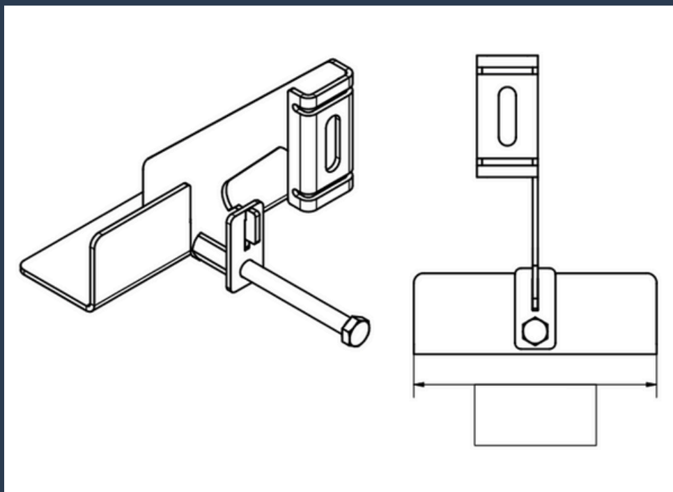
TSK-murkonsol type 3
