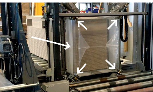
Der Prozess für Haubenstretchverpackungen
