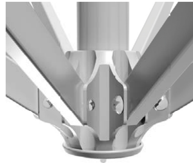
Hub for Amalfi PLUS – massive aluminum Centro de sombrilla Amalfi PLUS – de aluminio macizo
