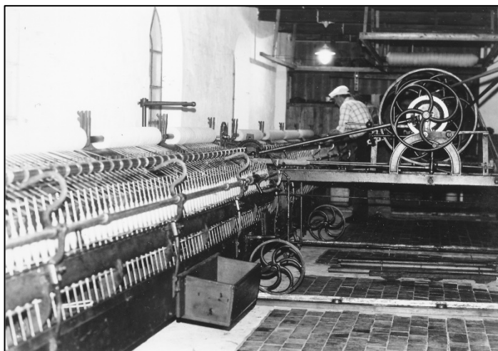
Spindemaskineri på Rebstrup Uldspinderi opstillet i Raadvad
