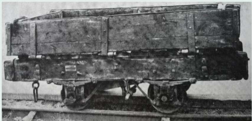
Öppen godsvagn använd på hästbanan Kristinehamn-Sjöändan 1850-1858. Foto Järnvägs-muséet, Gävle.
