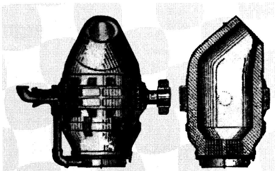
Bessemerkonverter:
