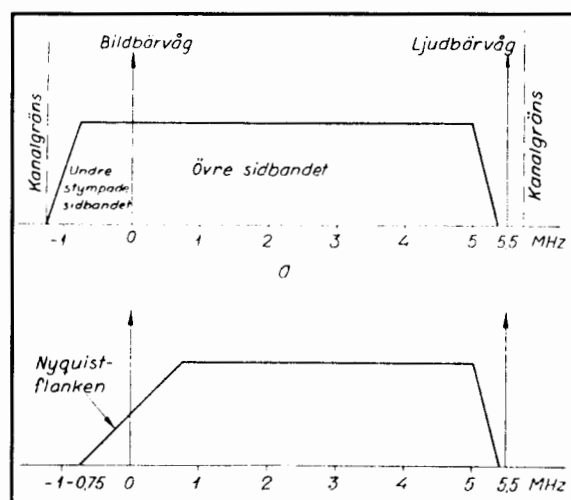
Mottagarkarakteristik för TV-mottagare. Ur James Hellström: TV-teknik
