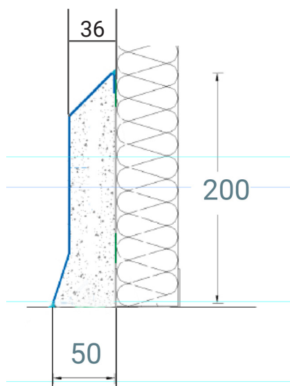
Indvendig hjørne
