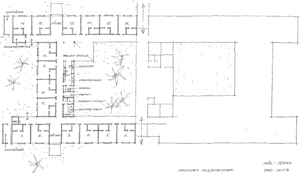
Ombygningsmodel B2
