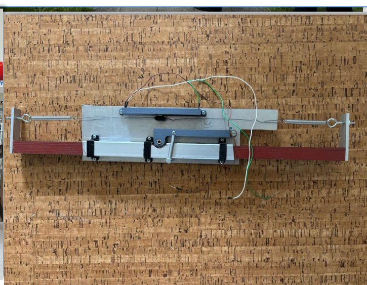
Stefan har konstruerat en ny bättre mekanism för pedalstyrningen på RB05 skjutsimulatore, som vi monterade på plats i kabinen.
