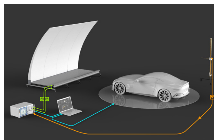
MIMO 2×2
