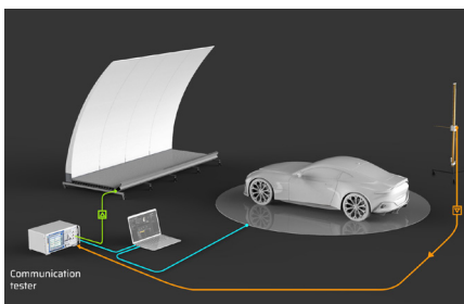
SIMO 1×2
