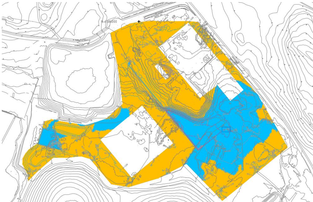
Figur 4-2: Områden där det behövs schaktning för placering av kvalificerad övertäckning. Områden som ska schaktas ur är markerade i gult, områden som ska fyllas är markerade i blått.
