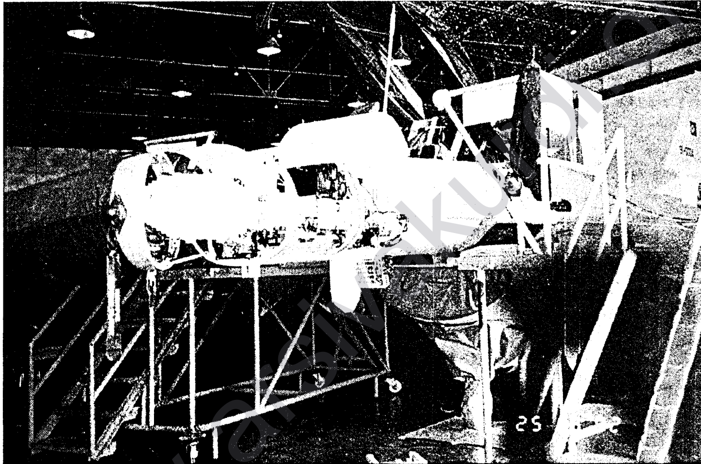
Besoin de sécurité : assemblage et fabrication d'avions F-16 dans les ateliers des Turkish Aerospace Industries, non loin d'Ankara. Photo « Le Soir ».
