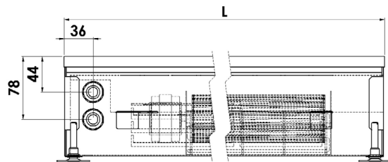
LONGITUDINAL SECTION
