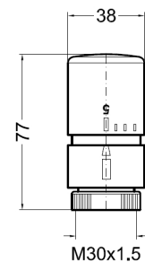
Tête thermostatique
