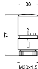
Tête thermostatique
