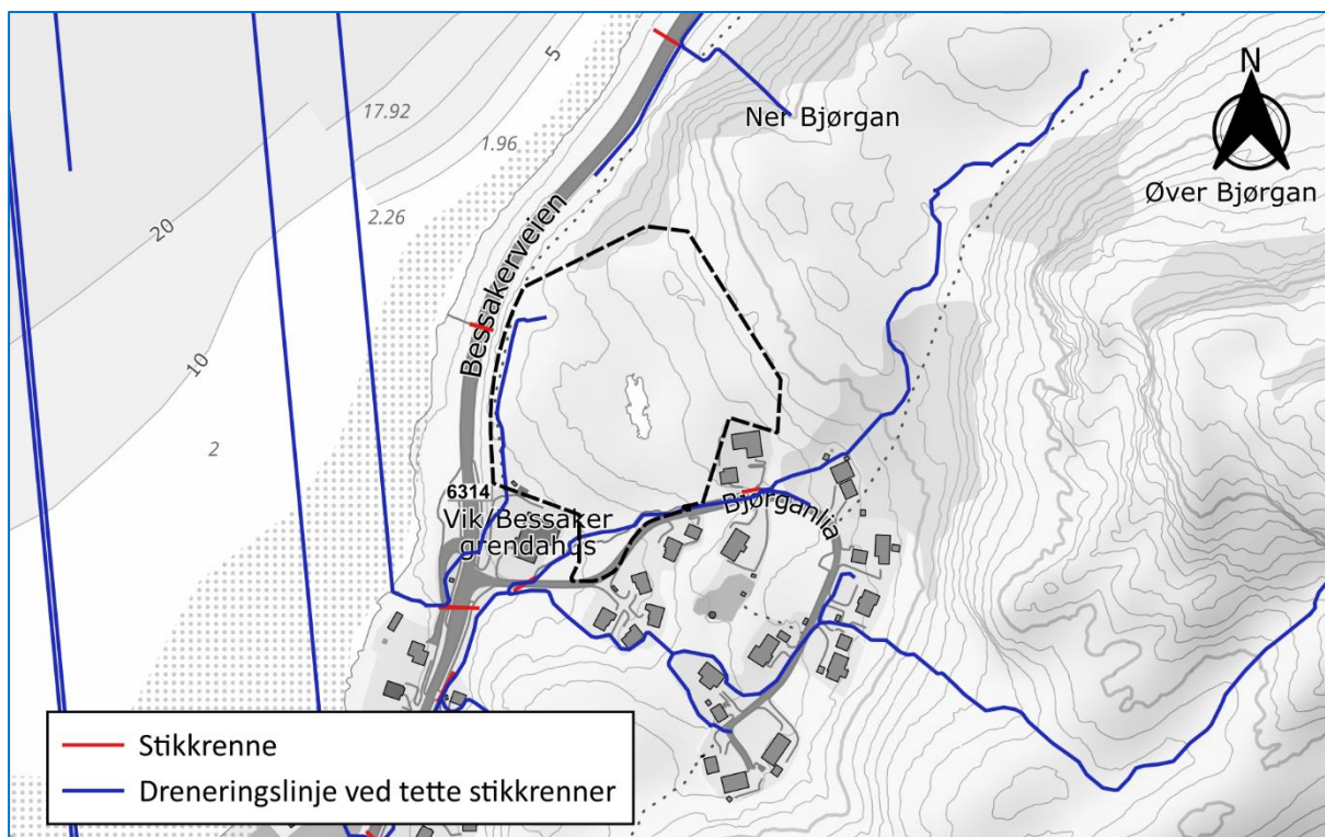
Figur 3 Overvannsproblematikk ved tette stikkrenner, M = 1:5 000.
