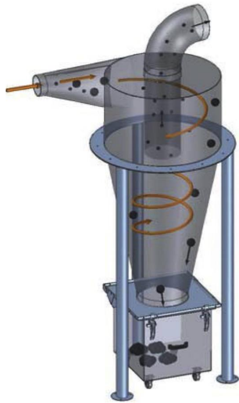
Separador ciclónico dibujo de funcionamiento
