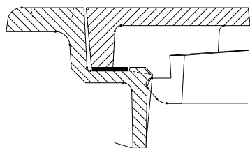
Detalj av lås
