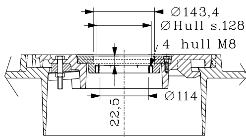
Detalj B:
