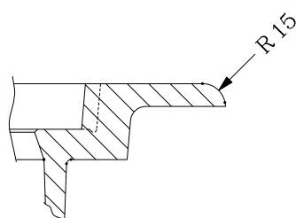
Detalj av flens
