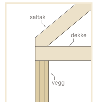
Snitt; møter mellom vegg, tak og dekke (i massivtre)
