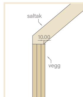
Snitt; møter mellom vegg, tak og dekke (i massivtre)
