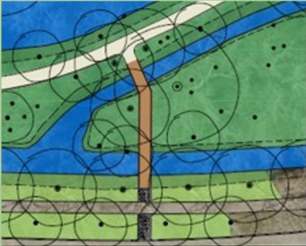
Ontwerp vloderbrug van bovenaf gezien
