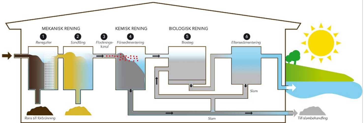
AVLOPPSRENINGSVERK
