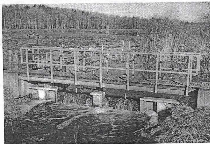
Dämmet i 30-meterskärret vid högvattennivå.
