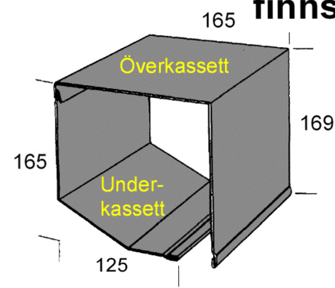
Kassett 165mm/90° överkassett Kassett 165mm/45° underkassett
