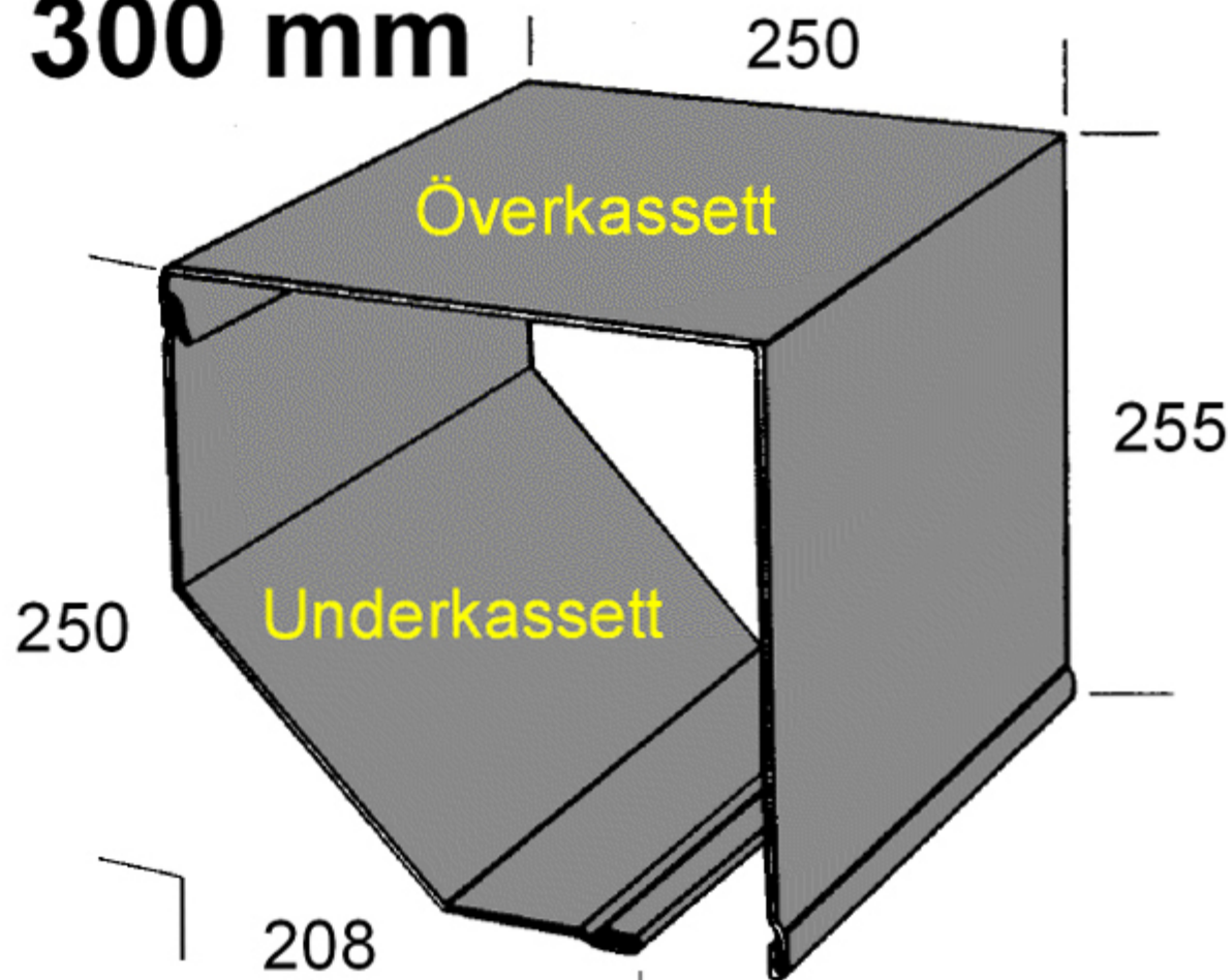
Kassett 250mm/90° överkassett Kassett 250mm/45° underkassett
