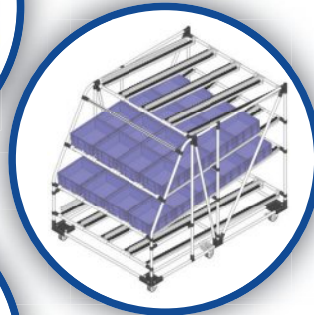
DURCHLAUFREGALE
