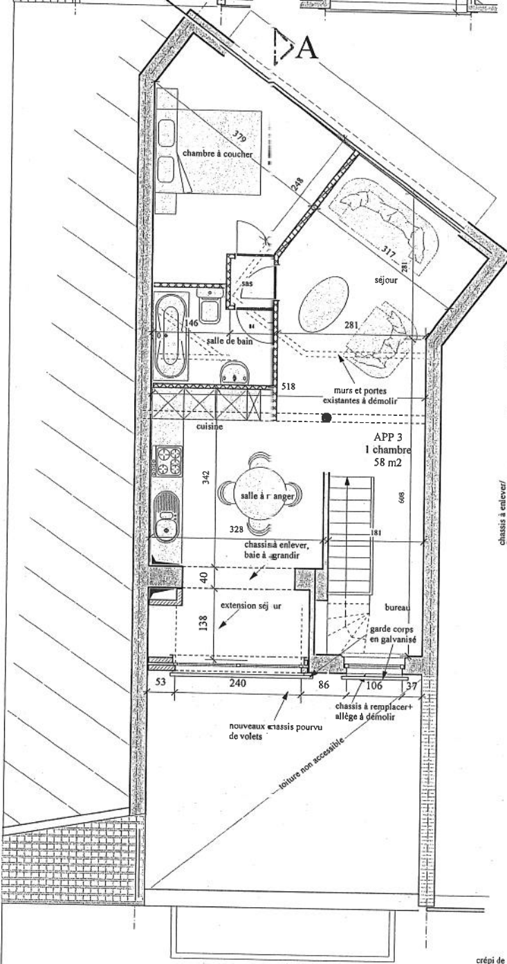
PROJET 3E ETAGE 1/50
