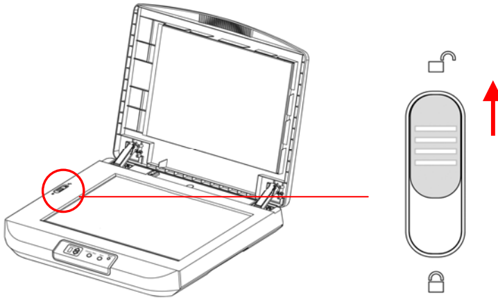
Abbildung 2-1 Transportsicherung entfernen
