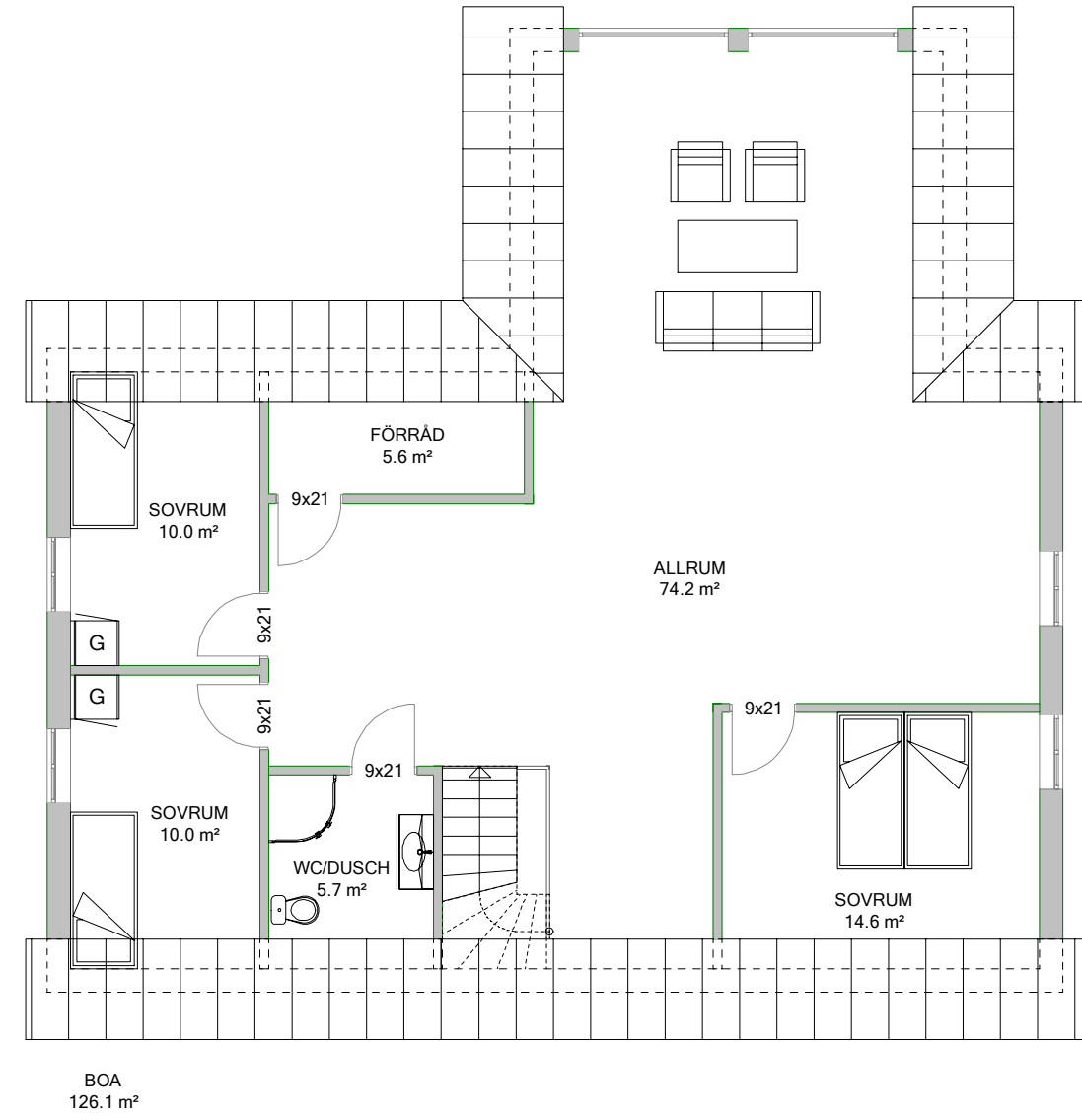
PLAN VÅN.2
