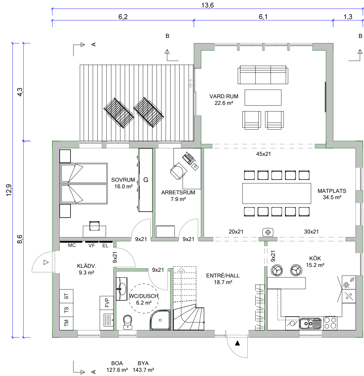
PLAN VÅN.1
