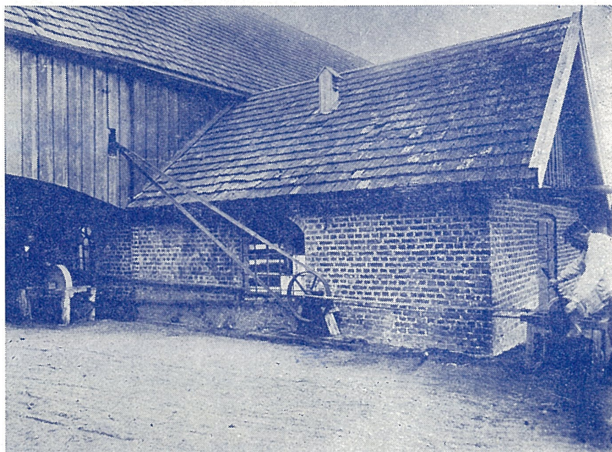
Den nye kraftkilden, elektrisiteten, tatt i bruk på gården Karlslyst i Hommelvik. Bildet er tatt ca. 1902, og viser to slipesteiner som drives av en elektrisk motor som er plassert på låven.
