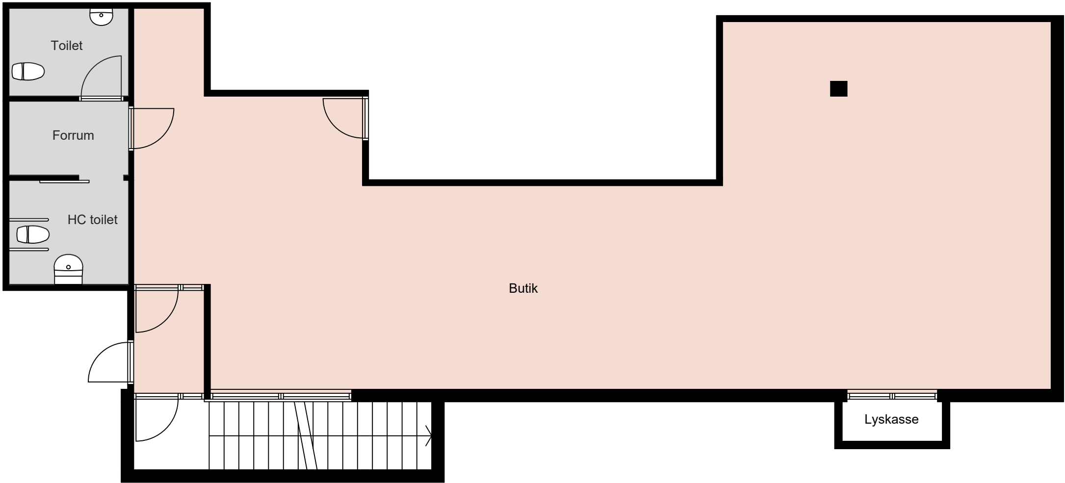
Kælderplan
