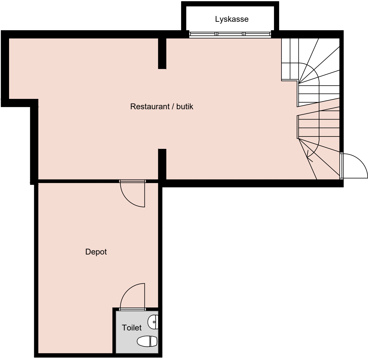
Kælderplan
