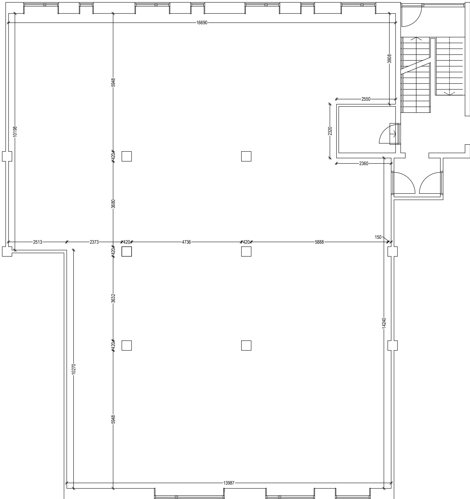
STUEPLAN, UDSNIT 1:100
