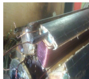
Rotoren i en 150KW generator under manuel omvikling
