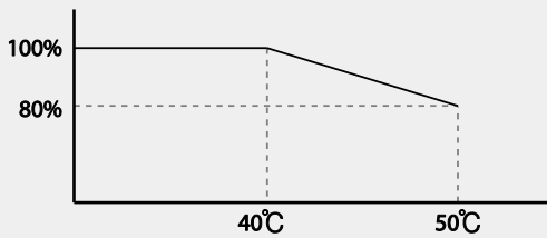
[Strombelastbarkeit als Funktion der Umgebungstemperatur bei normalem Lastmoment]
