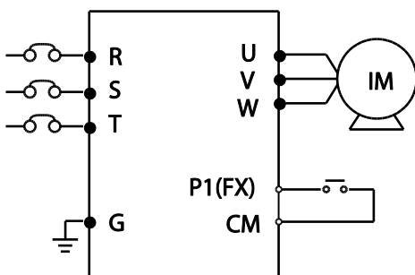
[Anschlussplan]
