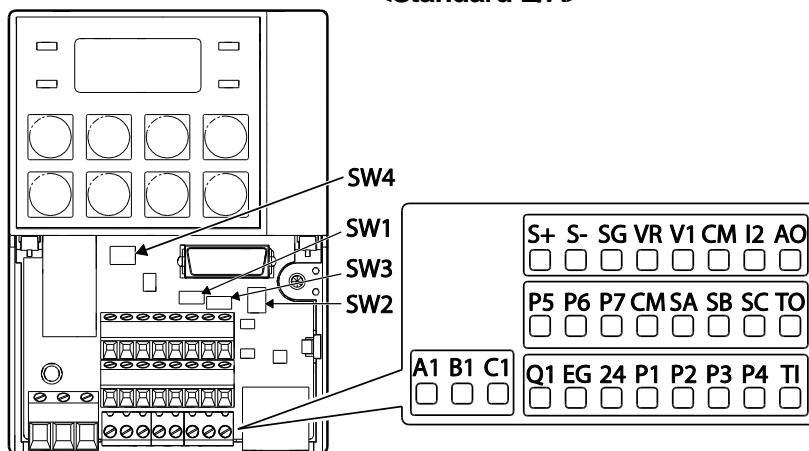
<Programmierbare E/A>
