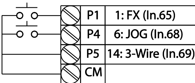
[Klemmenanschlüsse bei 3-Leiter-Betrieb]
