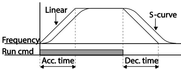
[Laufbefehl-Signalzustand und Beschleunigungs-/Verzögerungskurve]
