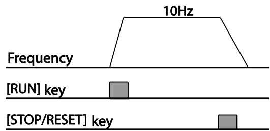
[Signalzustandsdiagramm]
