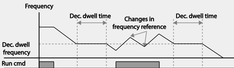
[Verzögerungsverweiloperation]
