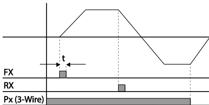
[3-Leiter-Betrieb]
