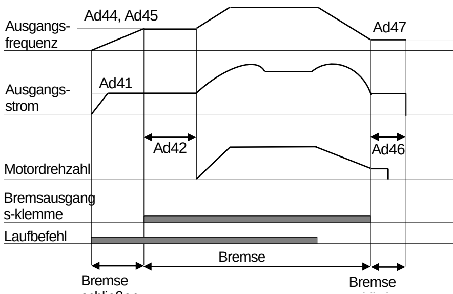
Lineare U/f-Steuerung
