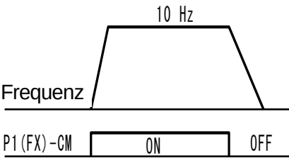
[Signalzustandsdiagramm]
