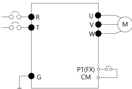
[Anschlussplan]
