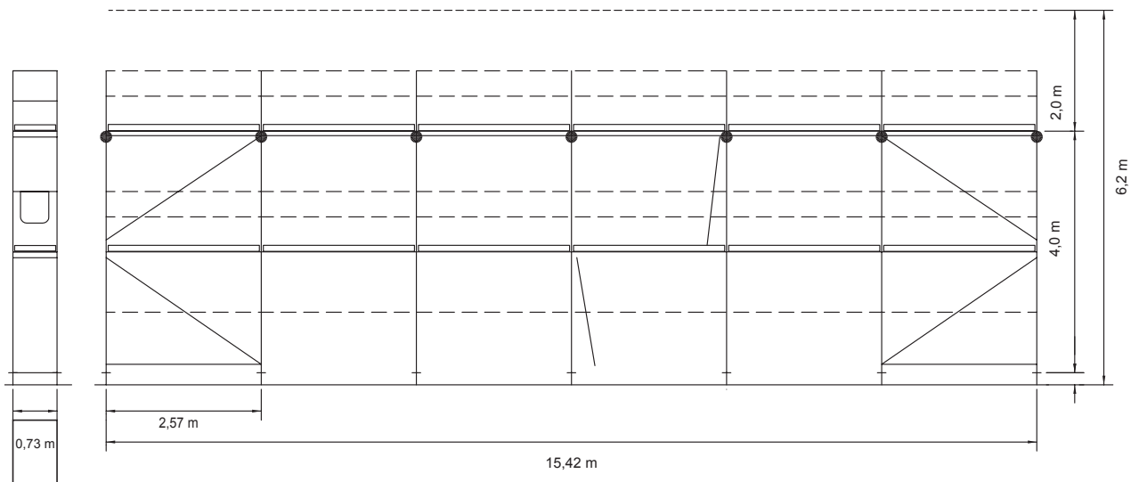
Gerüstbeispiel Feldweite 2,57 m ca. 96 m 2
