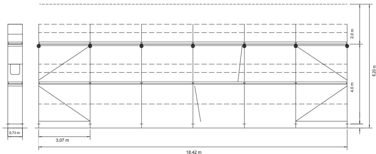
Gerüstbeispiel Feldweite 3,07 m ca. 115 m 2
