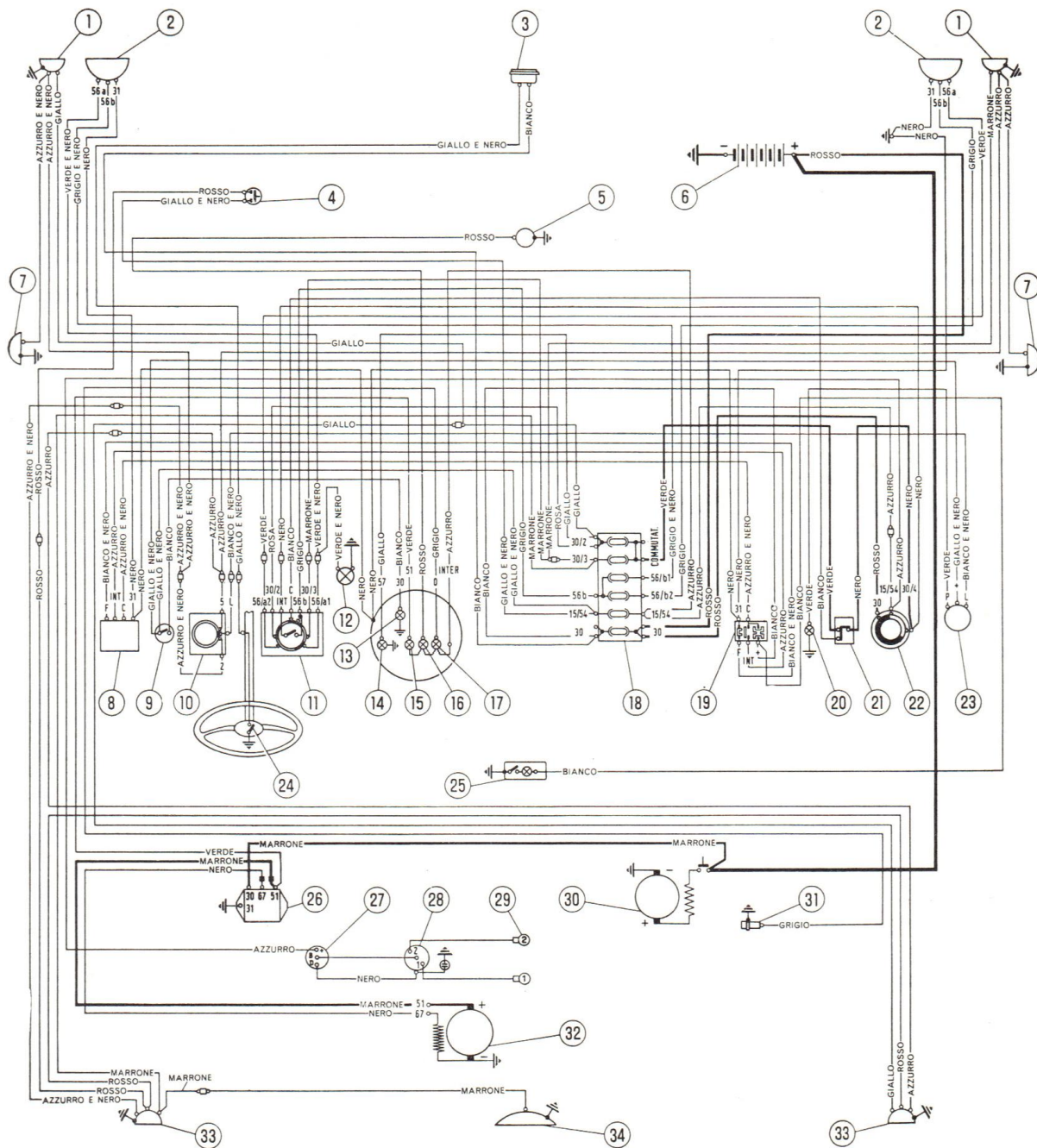
Fig. 54. Ledningsdiagram.
