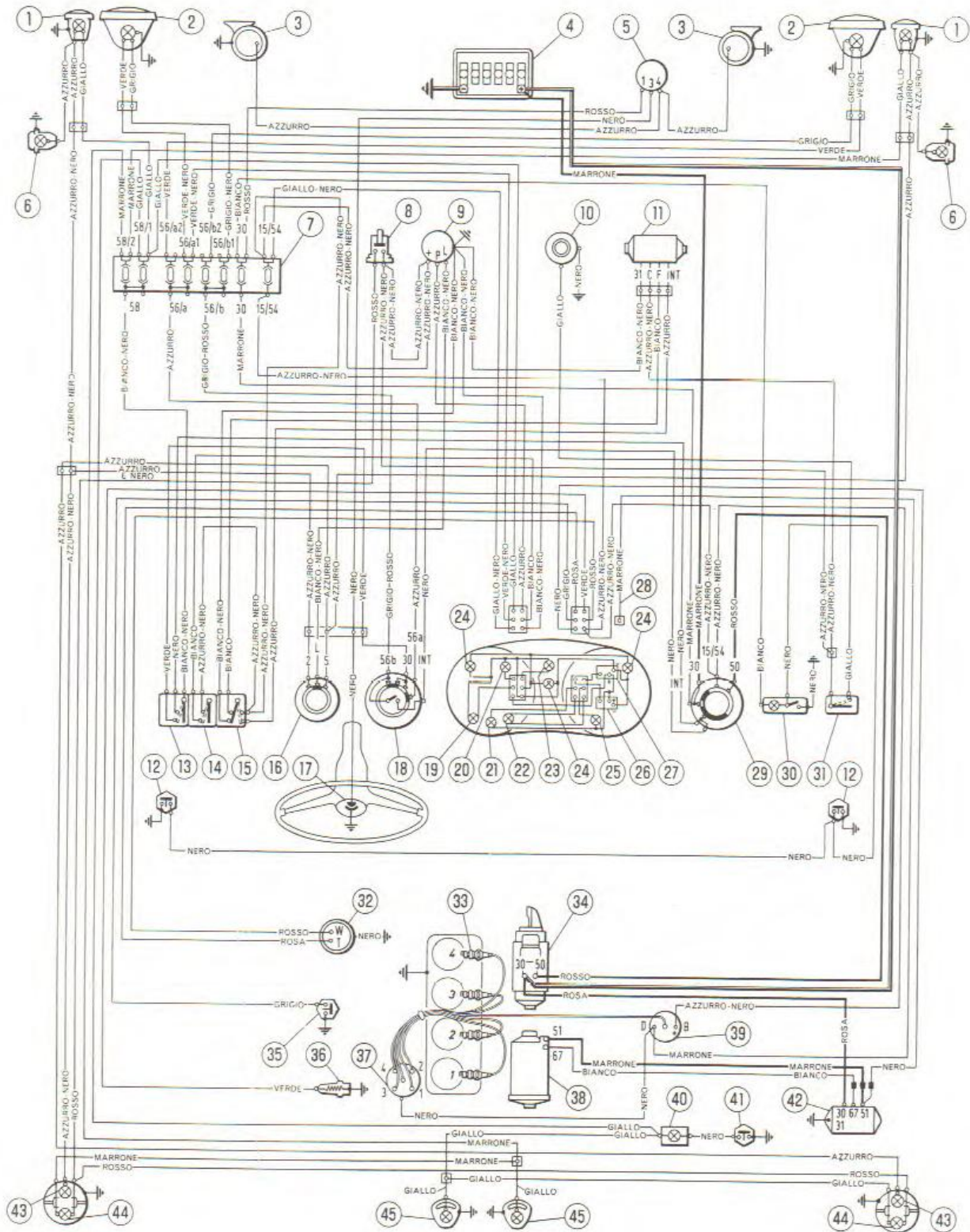
Fig. 46. Ledningsdiagram.
