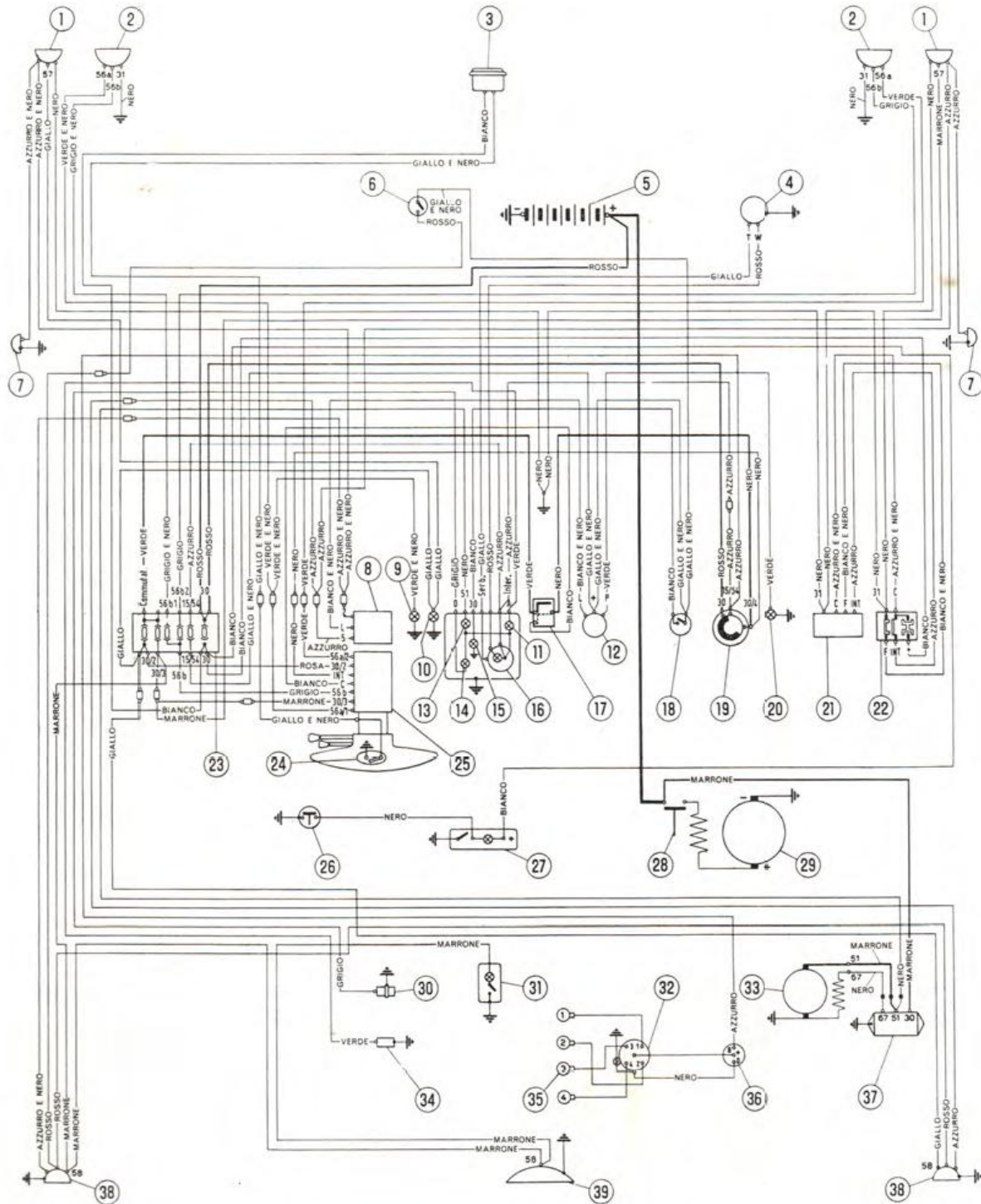
Fig. 51. Ledningsdiagram – Sedan.
