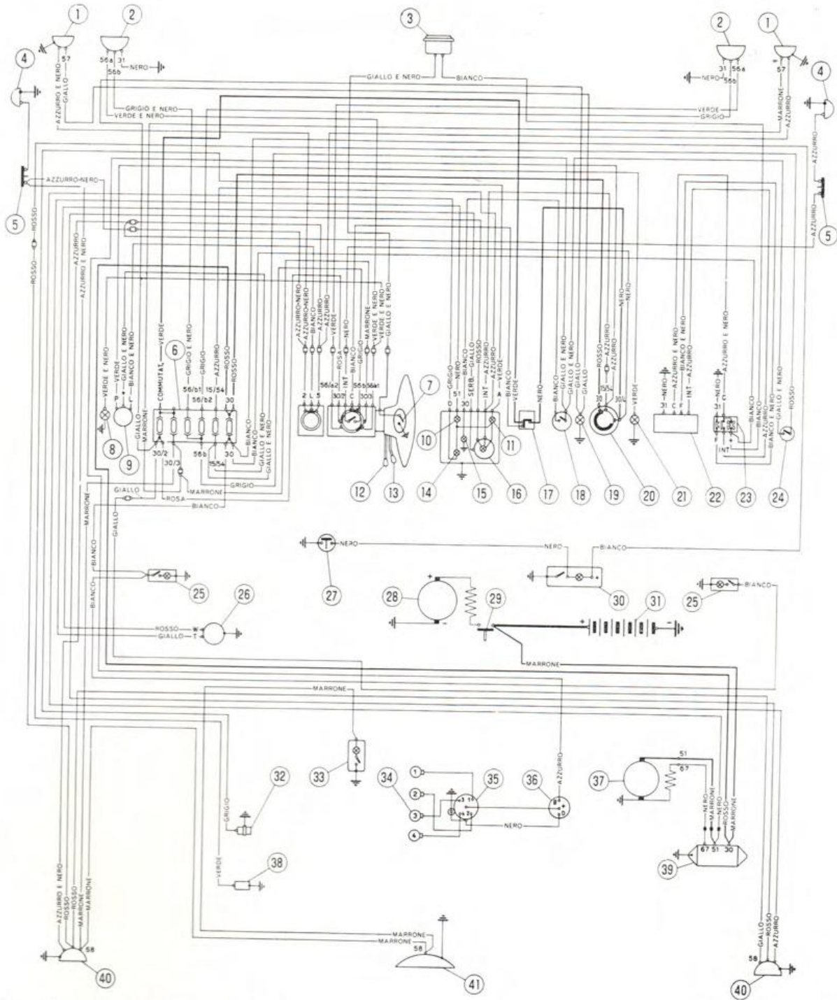
Fig. 52. Ledningsdiagram - Multipla.
