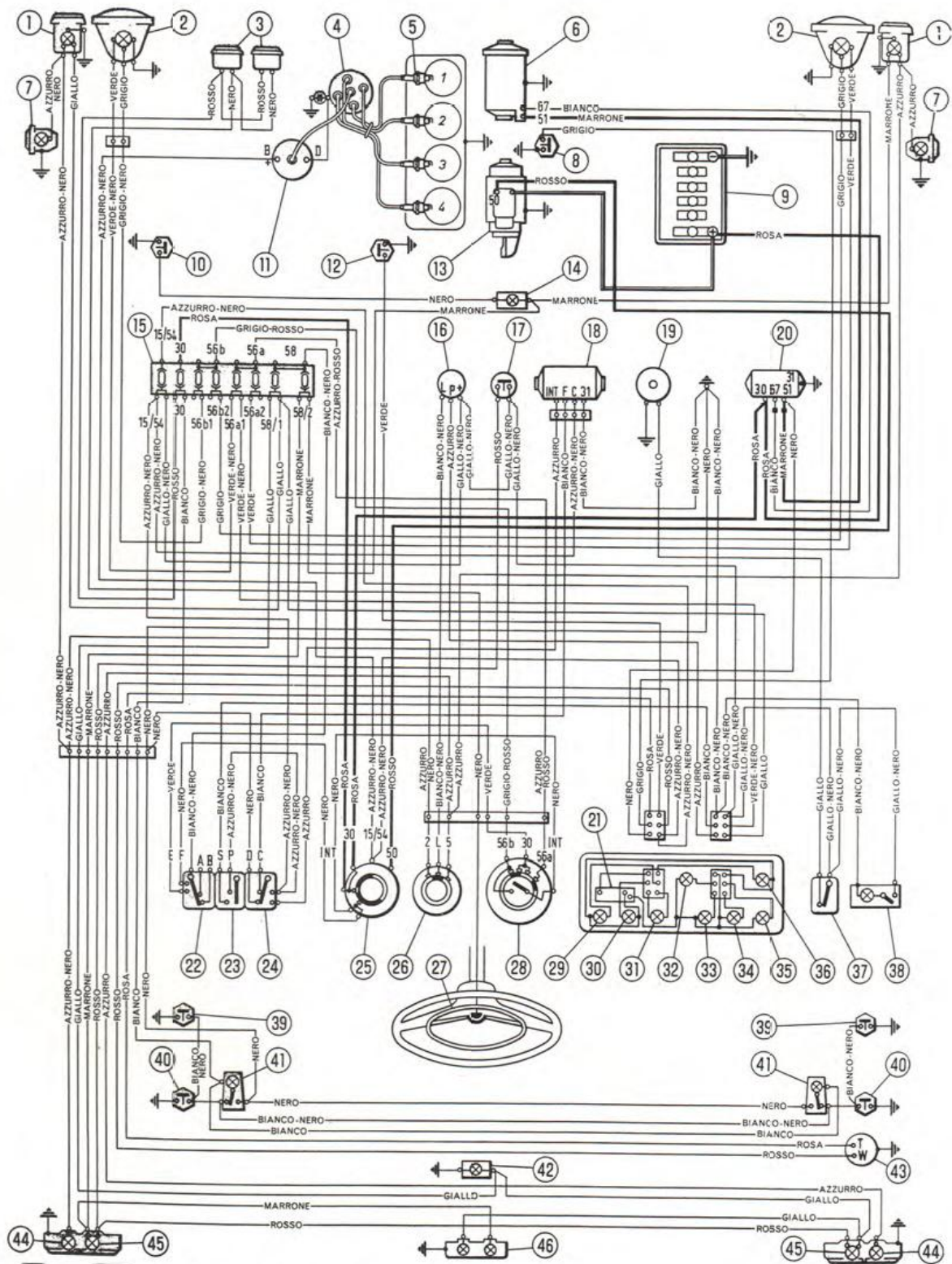
Fig. 53. Ledningsdiagram.
