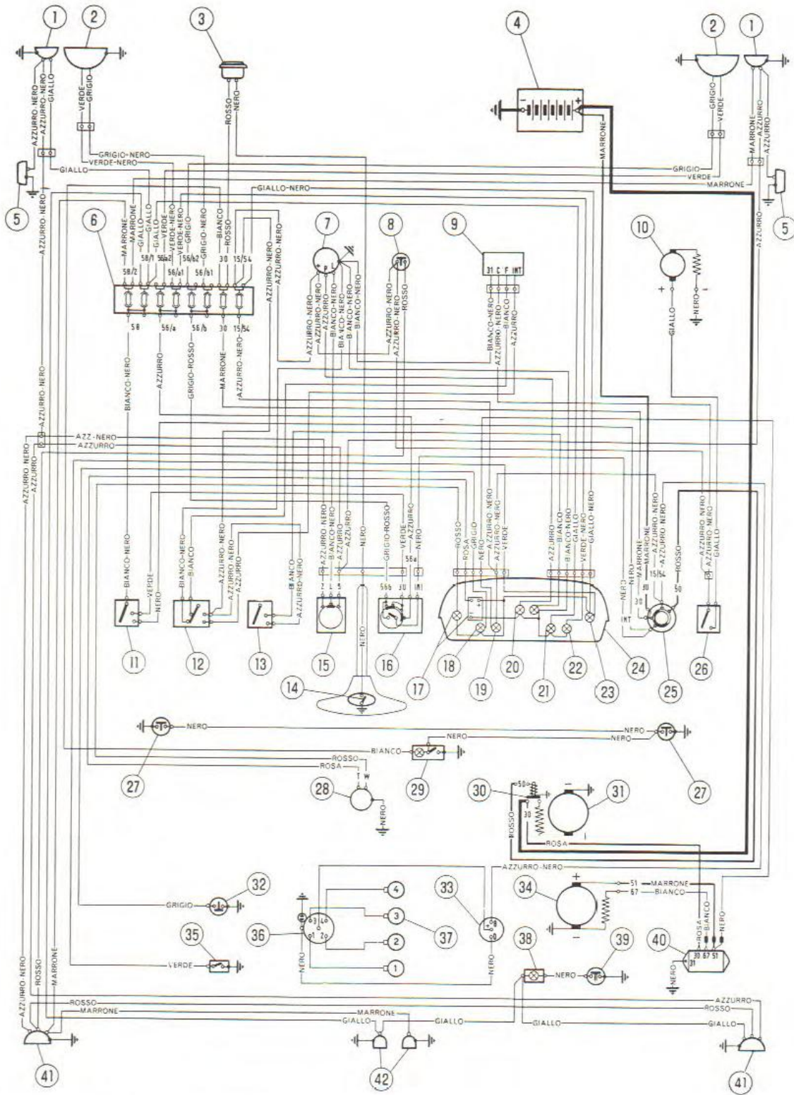
Fig. 53. Ledningsdiagram.
