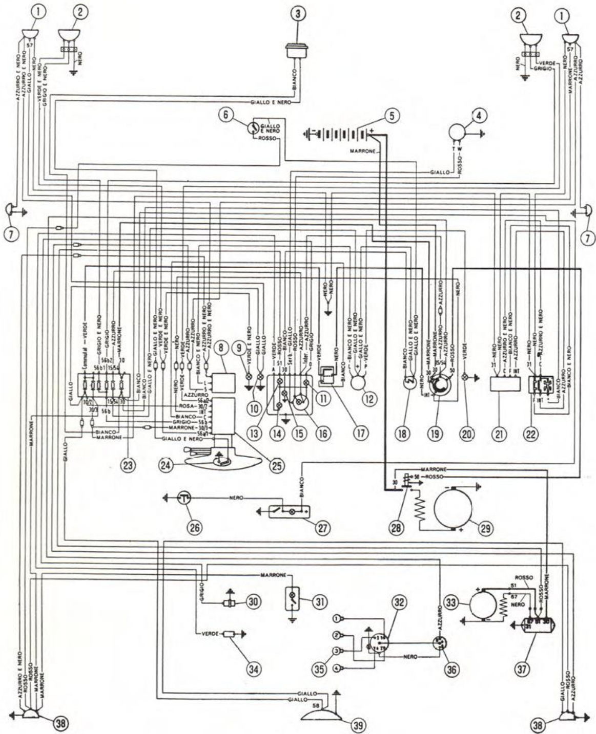
Fig. 41. Ledningsdiagram - 600 D Sedan.
