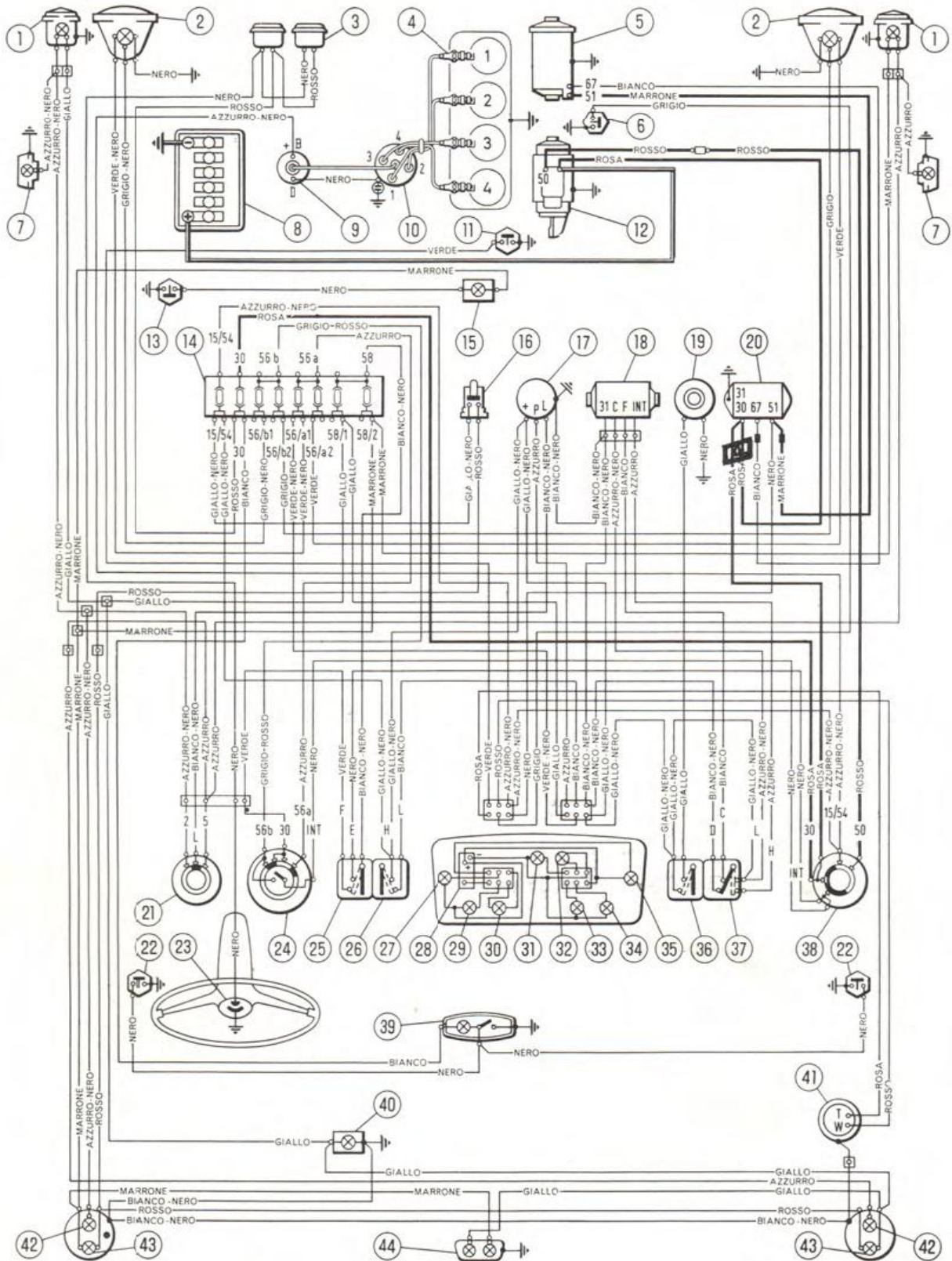
Fig. 36. Ledningsdiagram.
