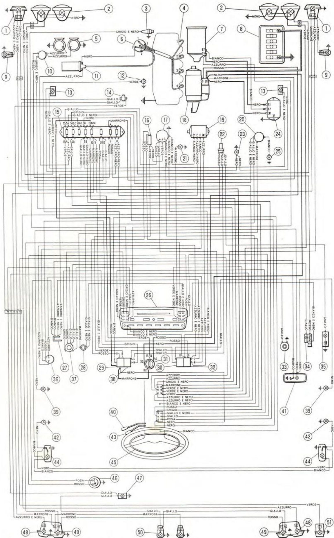
Fig. 49. Ledningsdiagram for FIAT 1300 og FIAT 1500.
