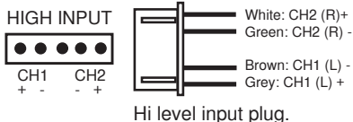
Hi level input plug.
