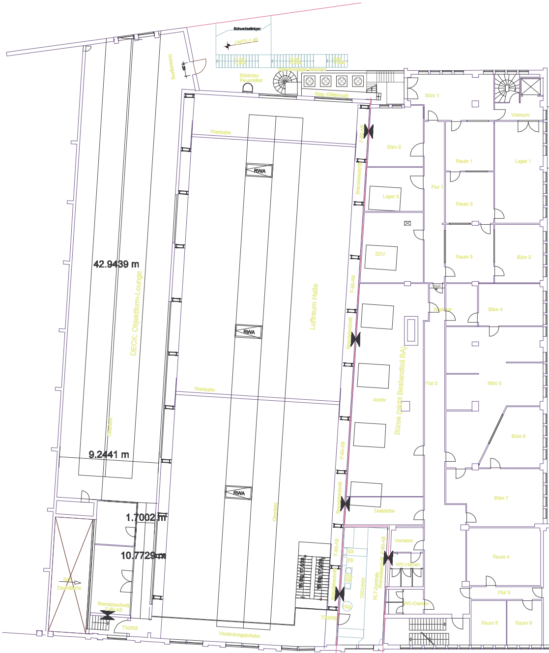
Grundriß Obergeschoß
