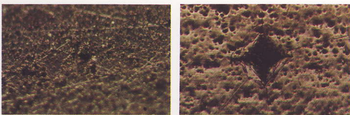
Mikrografischer (200x) Vergleich der Oberflächenfestigkeit einer Feinkernik- (links) und Aluminium- (rechts) Andruckplatte nach dem Aufschlag einer Diamantspitze mit einer Kraft von 1 kg.
