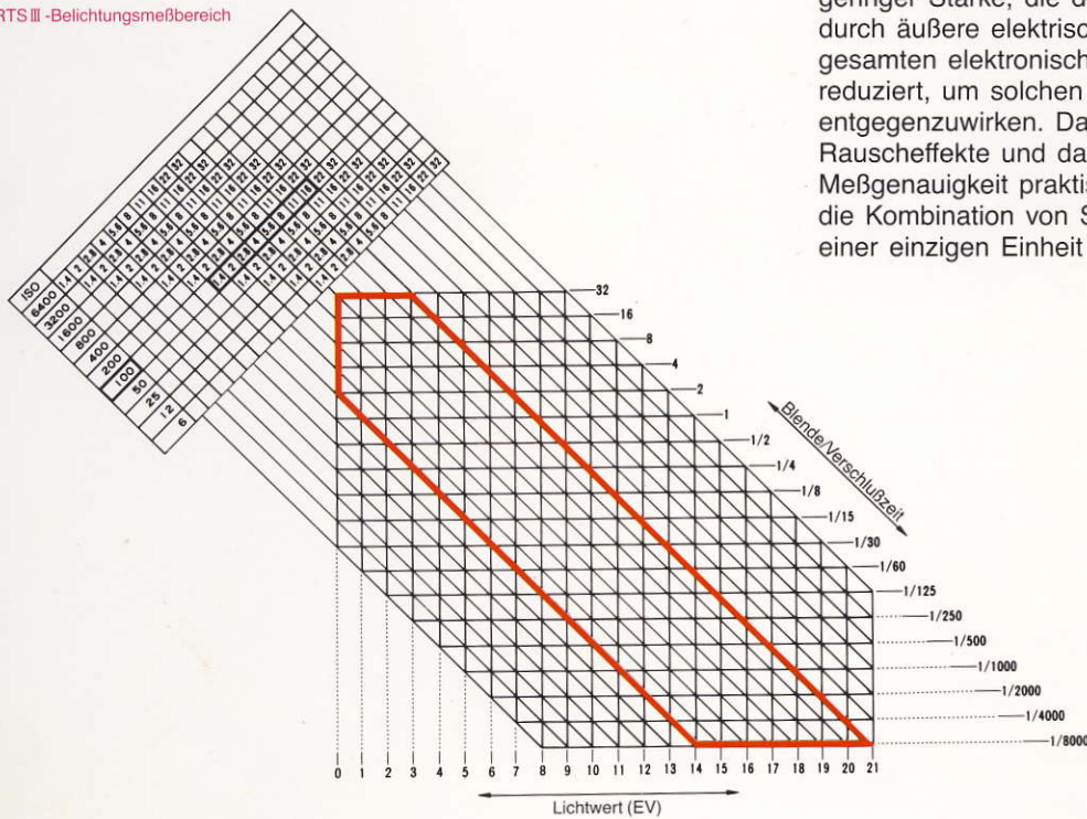
RTS III -Belichtungsmeßbereich
