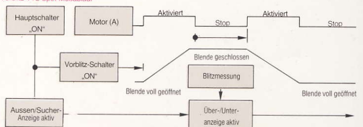
Vorblitz-TTL-Spot-Meßablauf
