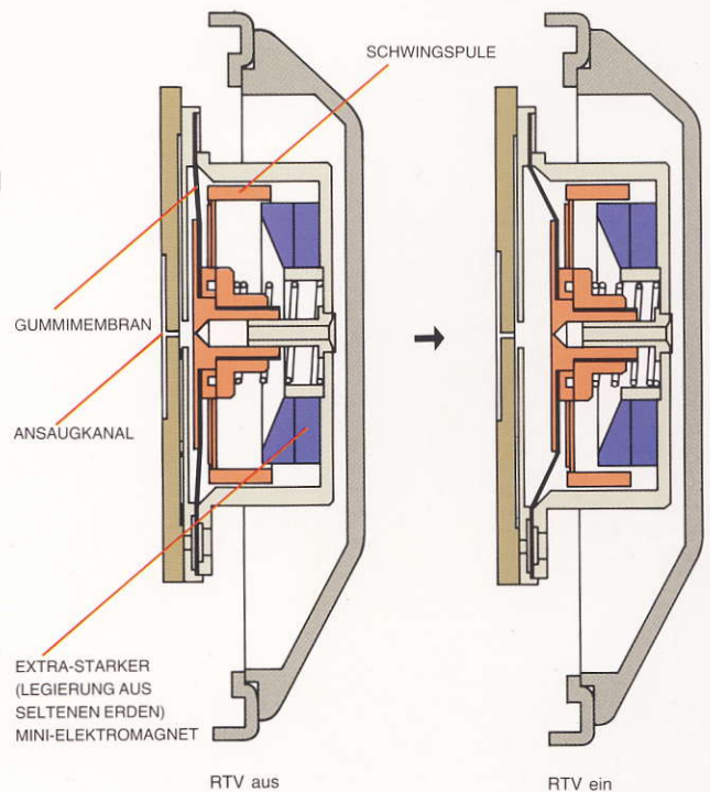
RTV SCHNITTZEICHNUNG
