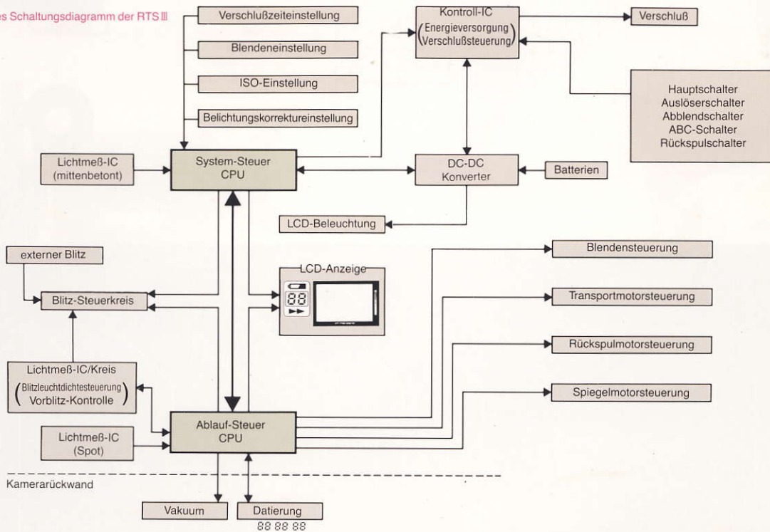
Elektronisches Schaltungsdiagramm der RTS III
