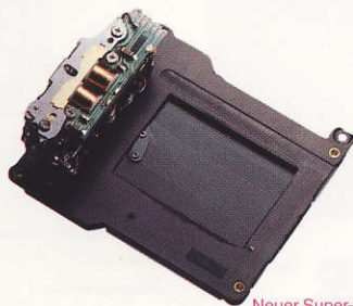
Neuer Super-Kurzzeit-Verschluss
