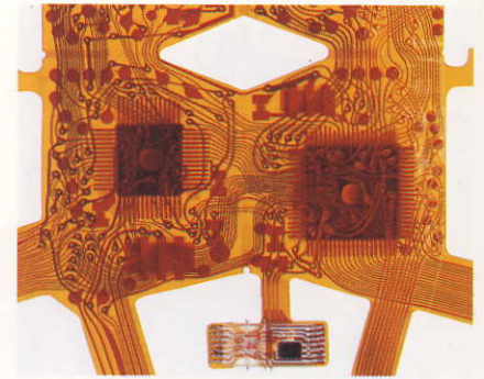
System-Steuer-CPU
