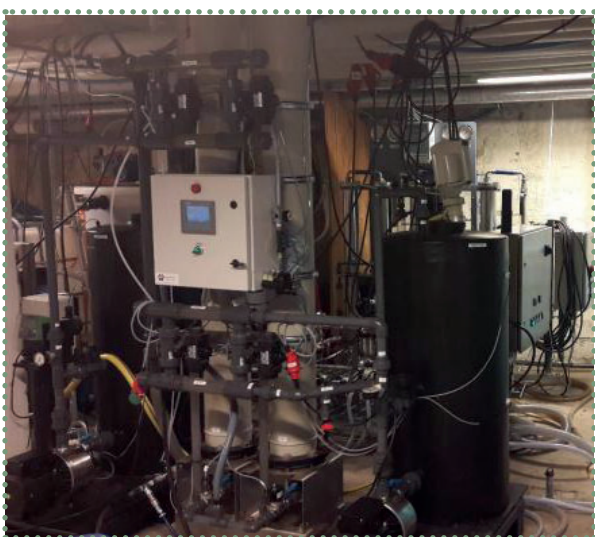
Aquadren's testanlæg hos Berendsen.
