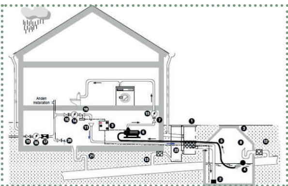
Skitseprojekt til håndtering af regnvand fra taget.
